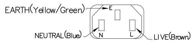
IEC 60320-1 C13
