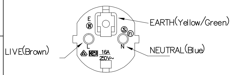
IEC 60884-1 CEE7-VII
