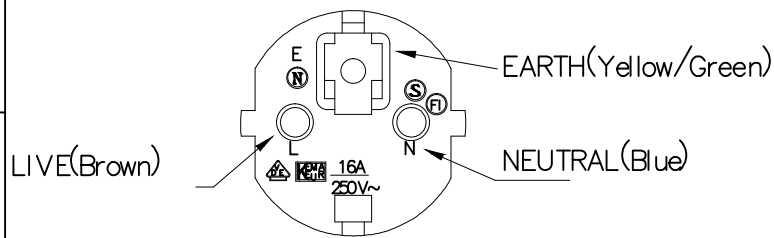
IEC 60884-1 CEE7-VII
