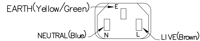
IEC 60320-1 C13
